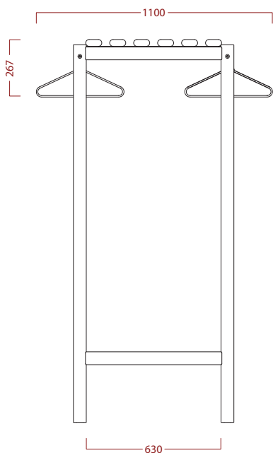
END ELEVATION
